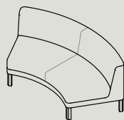
TB60 W 1595 D 1300 H 725 IR 1000 S400 W 62.8" D 51.2" H 28.5" IR 39.4" S 15.7"
