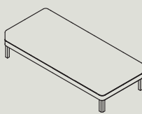
TO3 W 1800 D 770 H 400 W 70.9" D 30.3" H 15.7"
